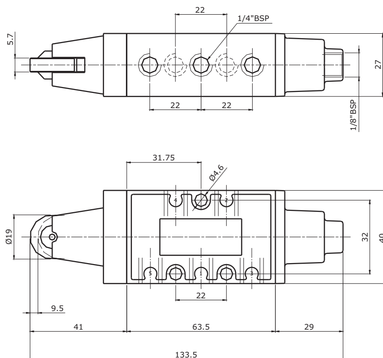
Válvula Rolete Piloto - 5/2 vias - Ref.: 20.5752-00
