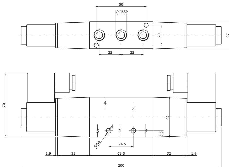
Válvula Duplo Solenóide - 5/2 vias - Ref.: 19P5882-XX
