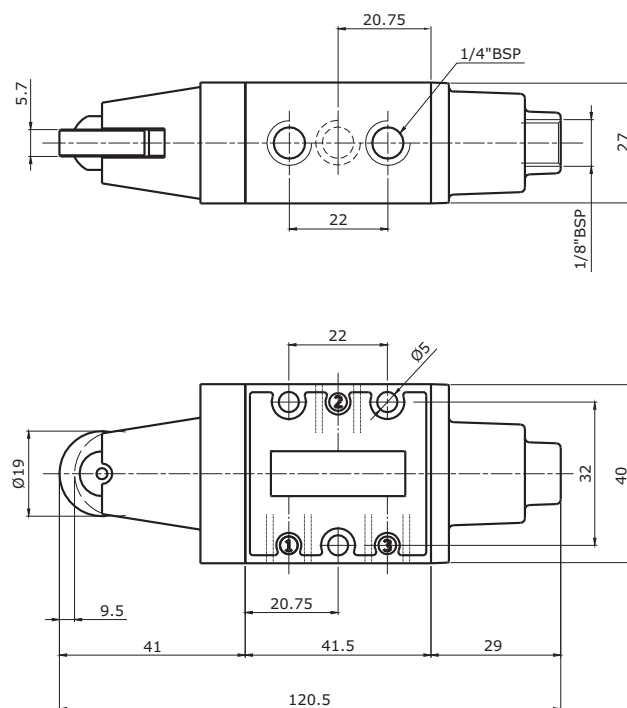
Válvula Rolete Piloto - 3/2 vias - Ref.: 20.3752-00
