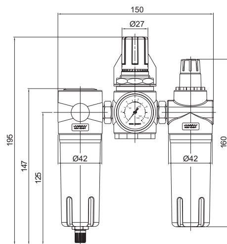
OPÇÃO COM COPO METÁLICO
