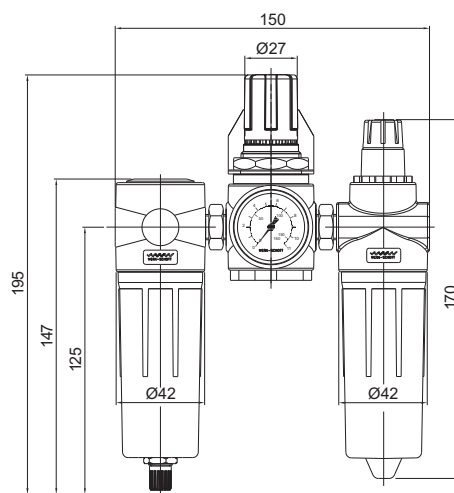
OPÇÃO COM COPO DE POLICARBONATO
